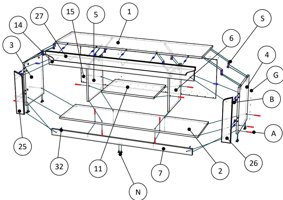
Рисунок 1. Сборка каркаса
