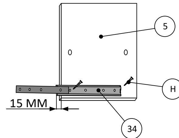
Рисунок 2. Установка направляющих
