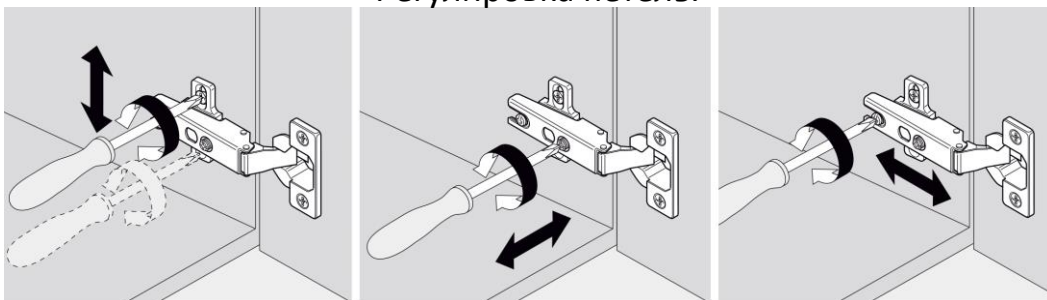
Регулировка петель.
