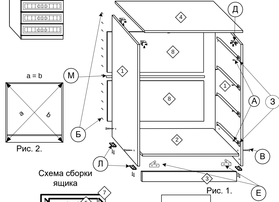
Схема сборки корпуса
