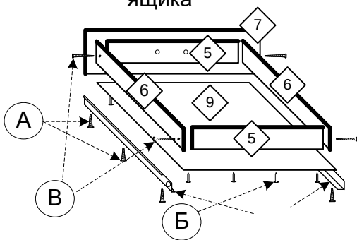
Схема сборки ящика
