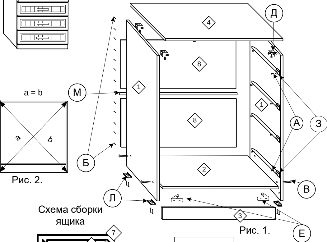
Схема сборки корпуса
