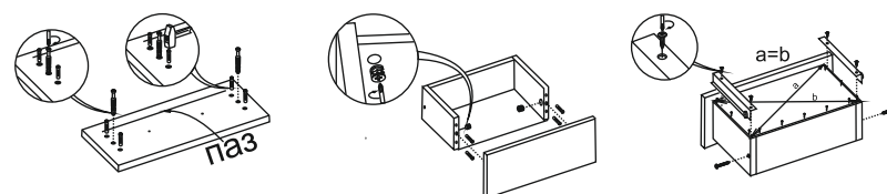
Порядок сборки выдвижного ящика
