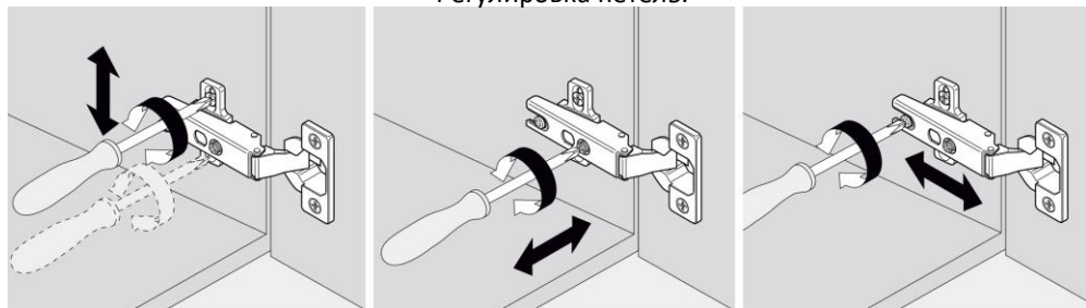
Регулировка петель.
